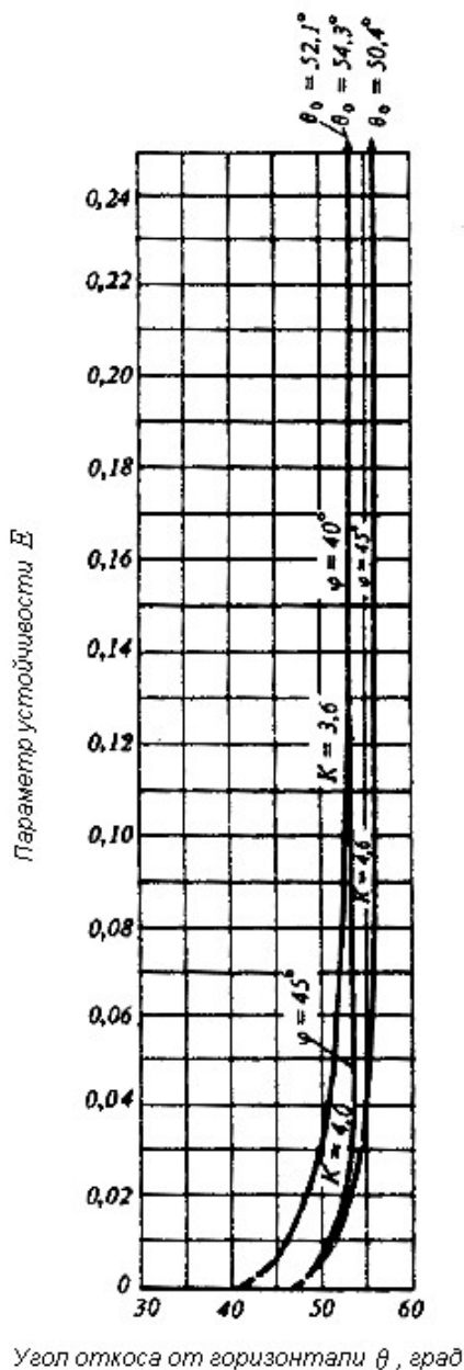
Черт.5. Графики для определения крутизны откоса при 3 < K \leq 5
